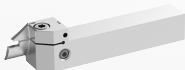
Porte-outil carré monobloc gorge frontale*
